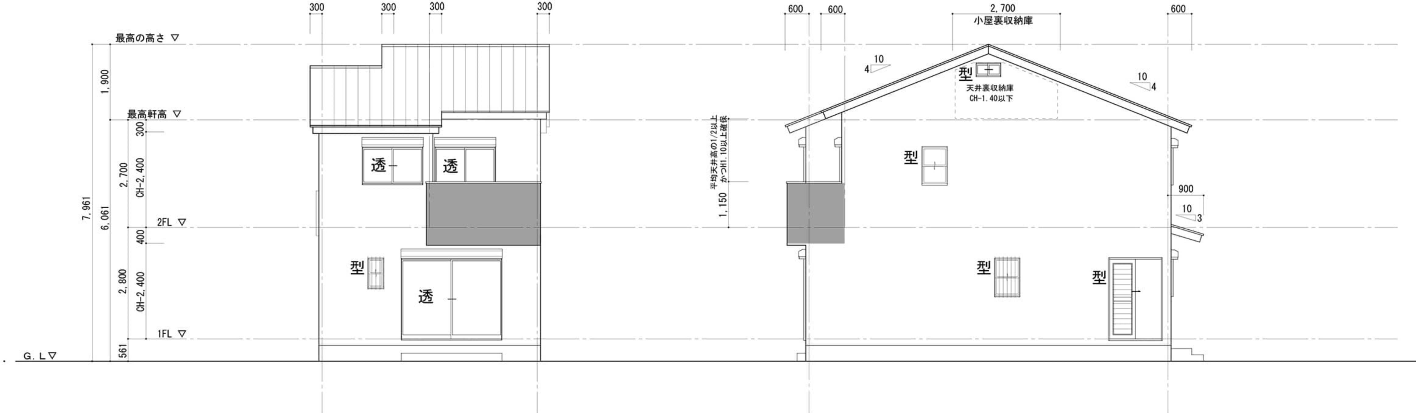
— 南 — 立 面 図
