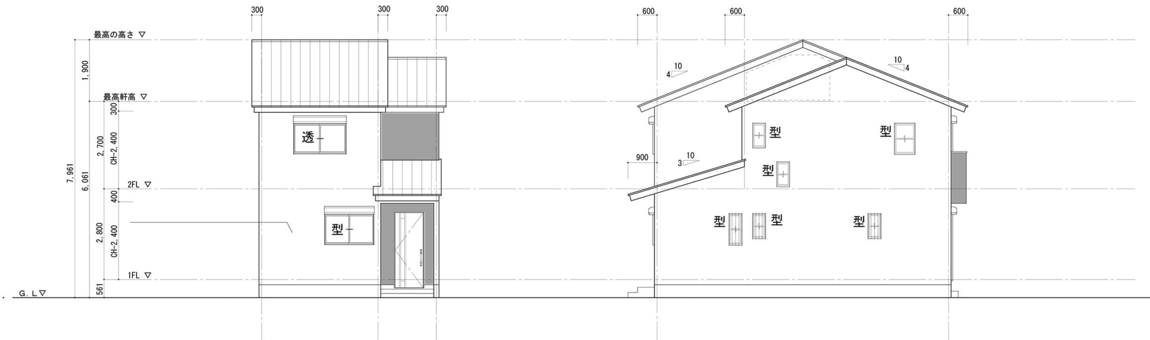
— 北 — 立 面 図
